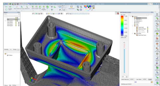
Análisis de desplazamiento
