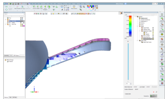
El modelo original, el modelo calculado y el modelo compensado (que se imprimirá para compensar el desplazamiento)
