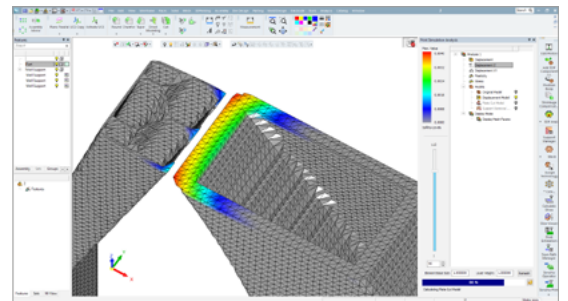
Análisis de interferencias del recubridor
