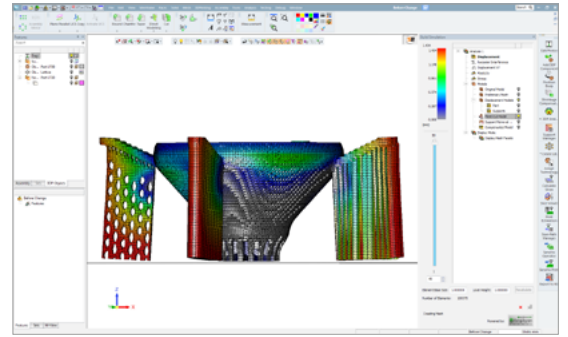
Deformación de diferentes tipos de soporte después de recortarlos de la placa
